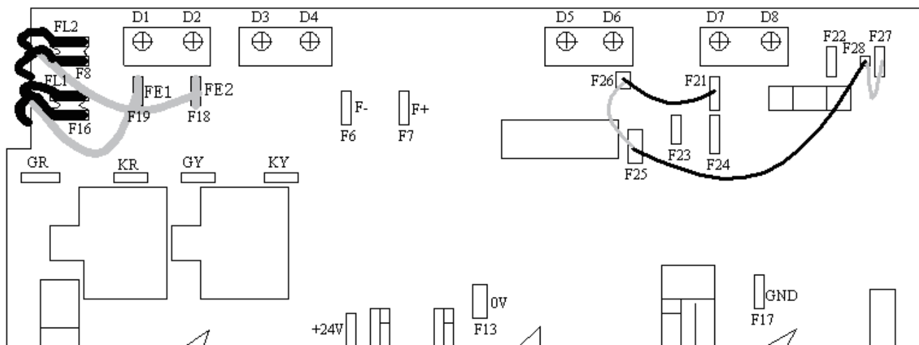
图 29 励磁接线转换
