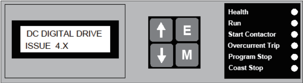
图 33 面板键盘
