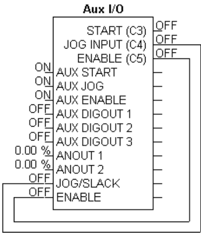
图 25 辅助 I/O功能块
