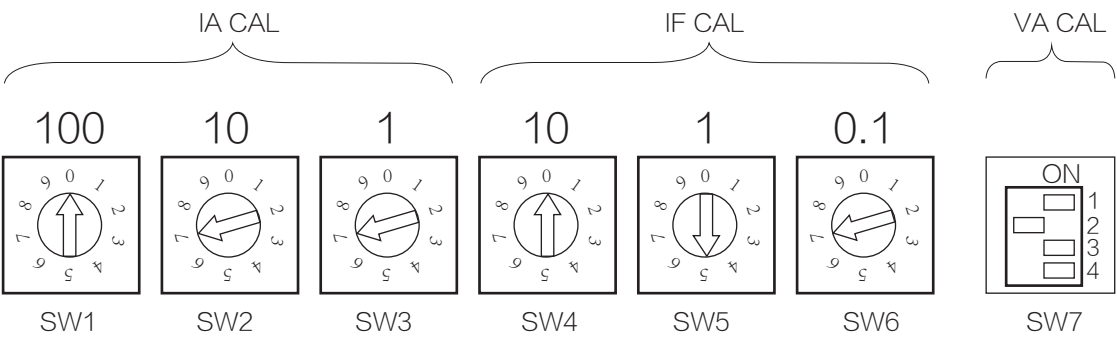
图 11 校准设置
