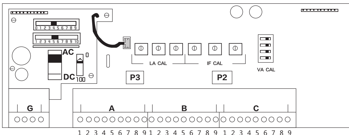
图 13 控制端子
