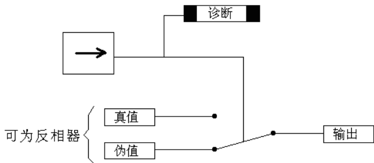
图 24 数字输入逻辑图
