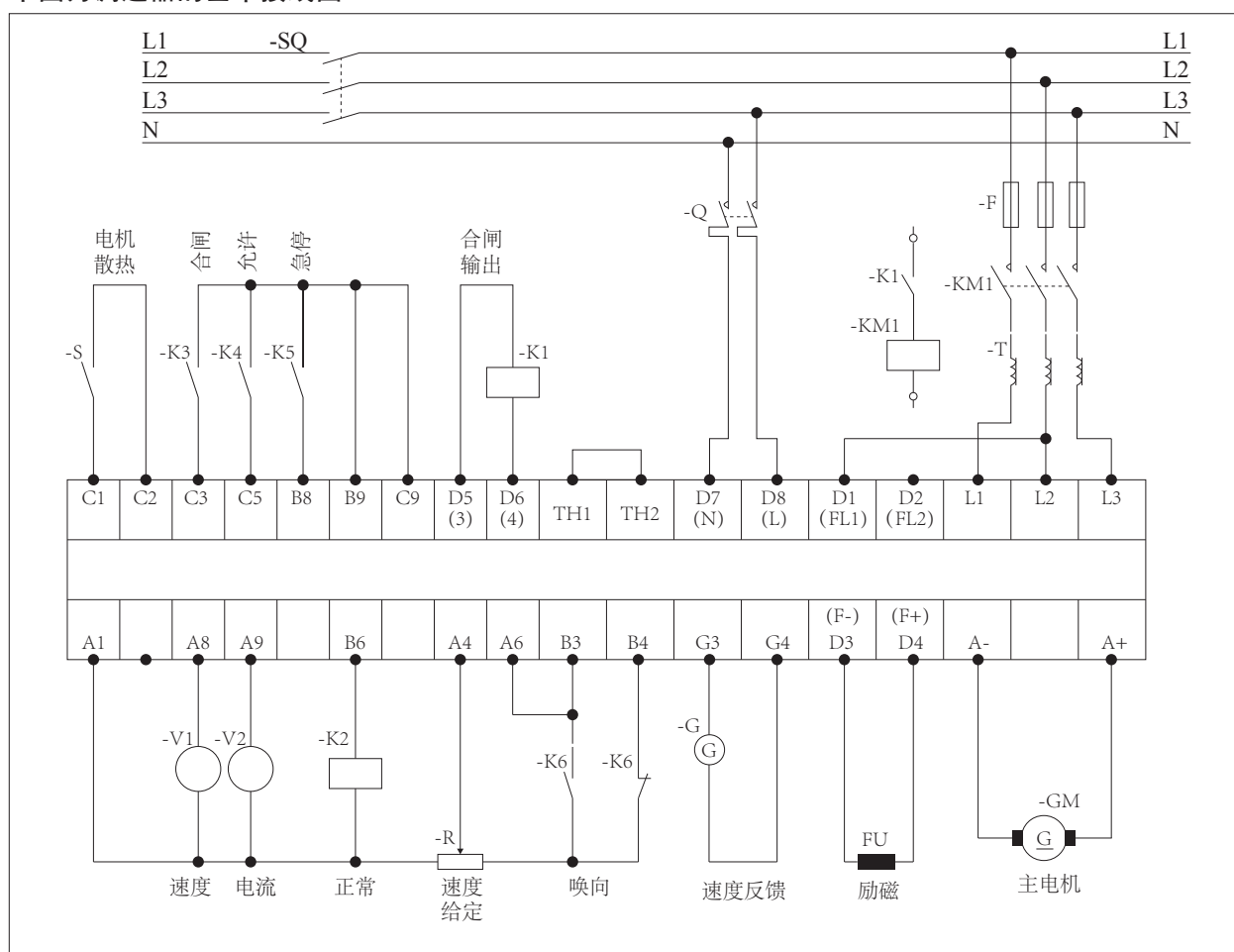
图 10 基本控制原理图
